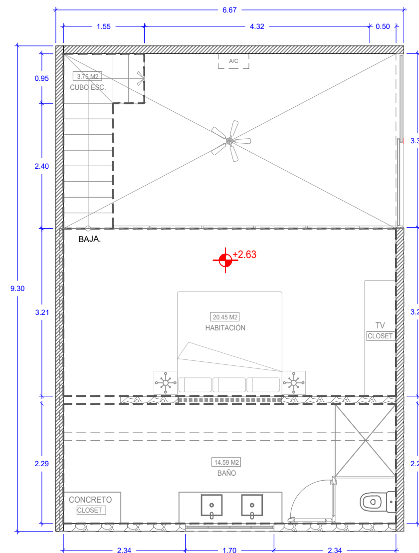
PLANTA TIPO LOFT 3 (D) - 38.27 M2 ESPESOR MUROS 15CM - (3.23 M2)
