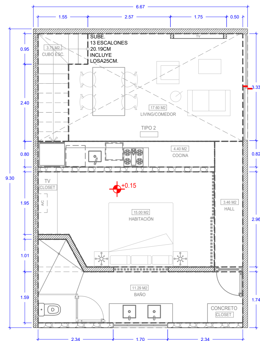
PLANTA TIPO LOFT 3 (D) - 61.36 M2 ESPESOR MUROS 15CM - (5.86 M2)
